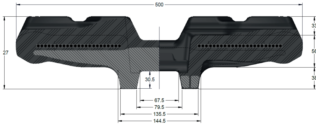
QUERSCHNITT
